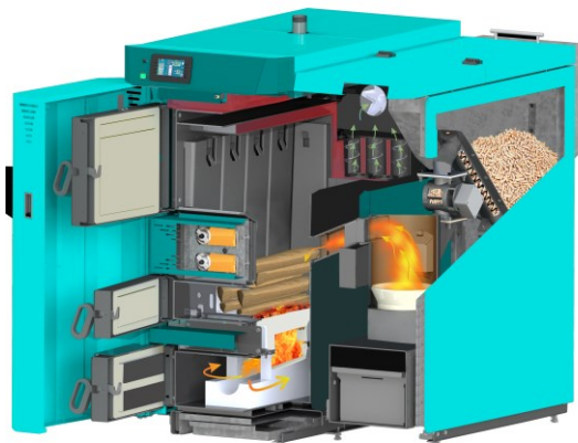
Schnittbild
